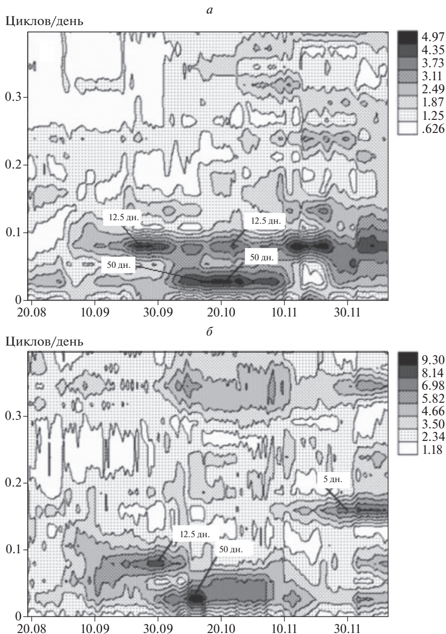
Рис. 4. СВД-диаграмма температуры ( a ) и влажности ( б ) для ГМС Горно-Алтайск.
