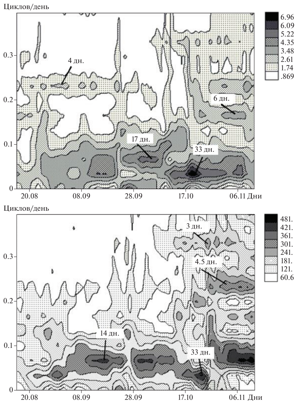
Рис. 8. СVAN-диаграмма температуры и давления в эпицентральной области Чуйского землетрясения.
